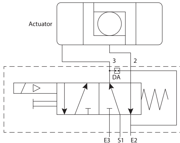
Fig. 2 Válvula pneumática de retorno da mola com piloto duplo no atuador de dupla ação com o circulador fechado
